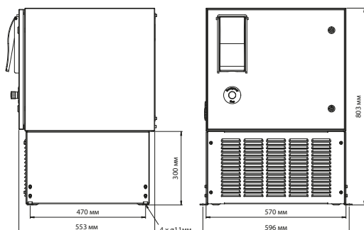
Стационарная установка
