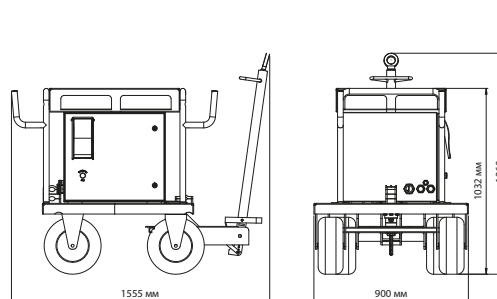
Мобильная установка*
