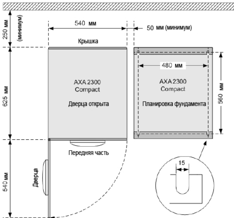
Рис. 4.4.1. Занимаемая агрегатом площадь, стационарная модель
